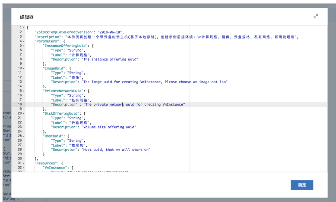
图 5: 展开编辑器
