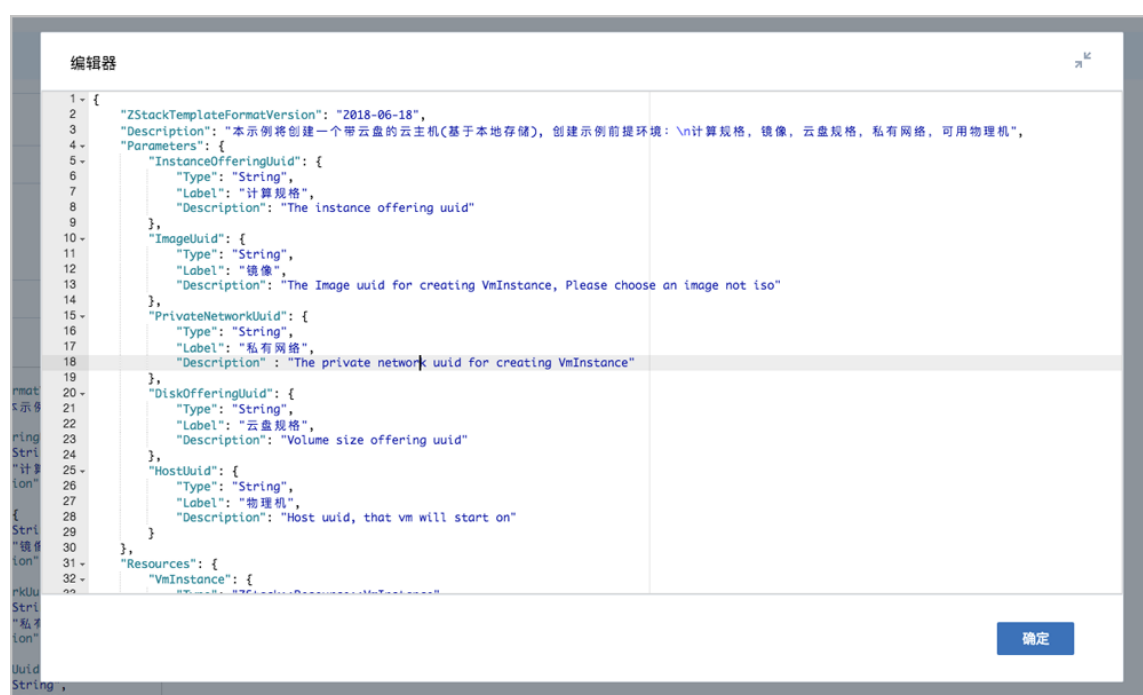
图 9: 展开编辑器
